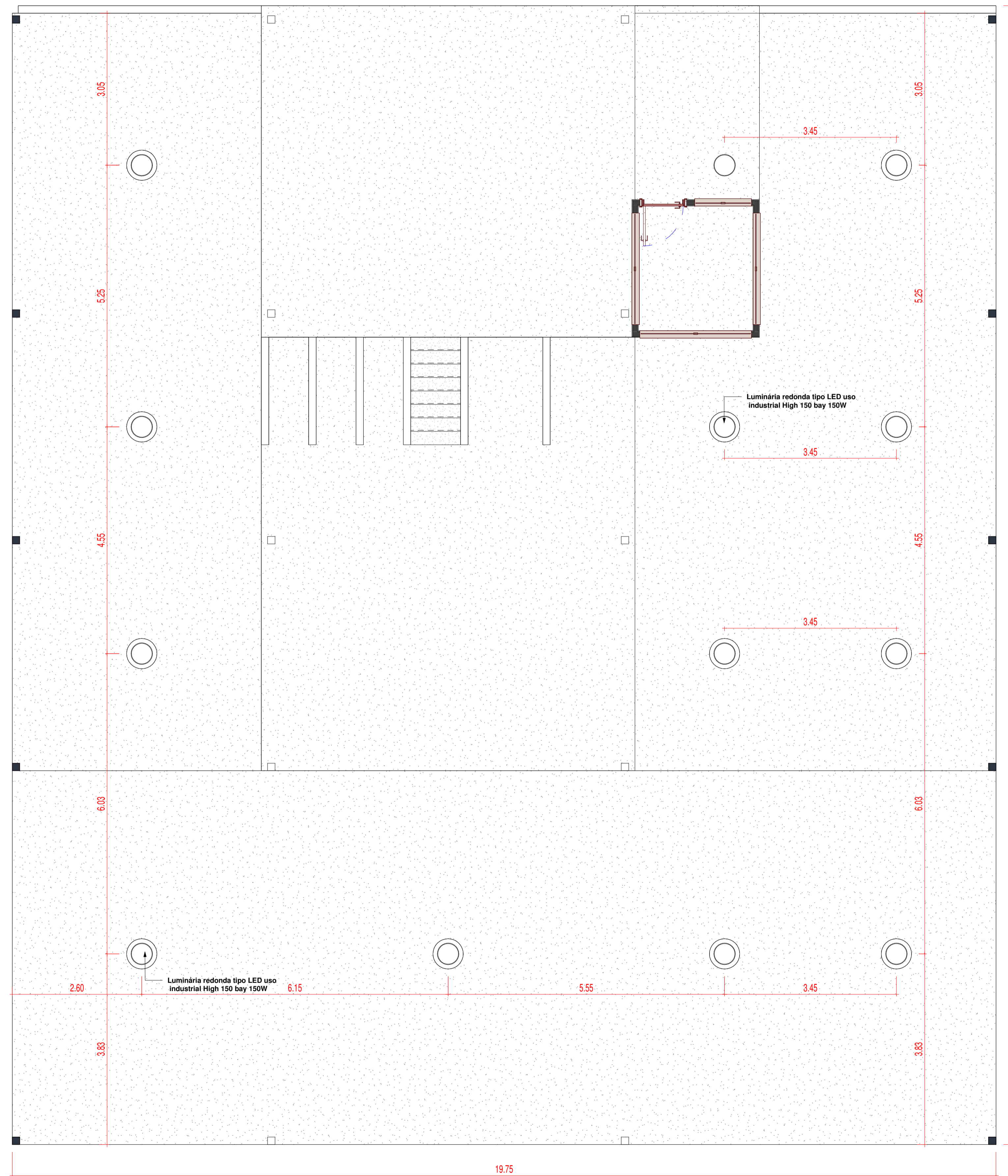
1 PONTOS DE ILUMINAÇÃO 1 : 50
